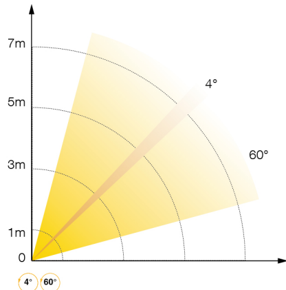
Light Output (FC=LUX × 0.0929)
